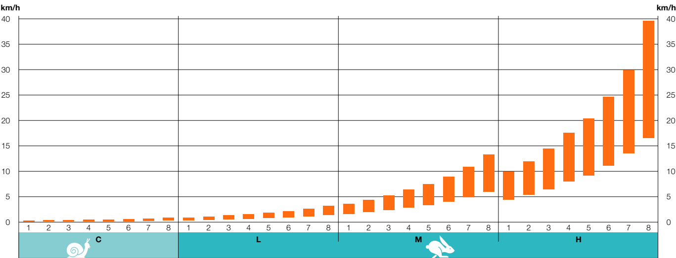
Speeds M6-121 U, M6-131 U, M6-141 U
